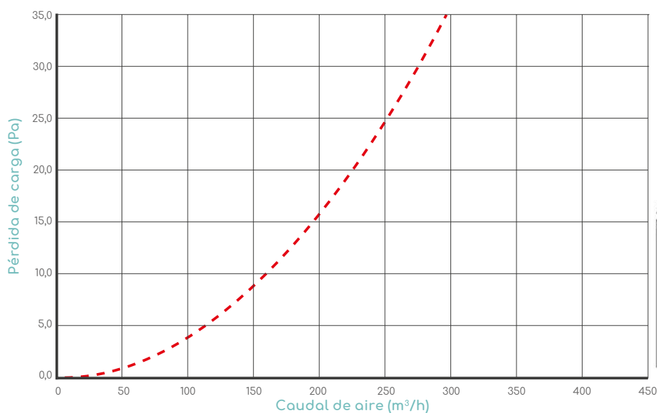
Pérdida de carga - Distribuidor completo 7x75
