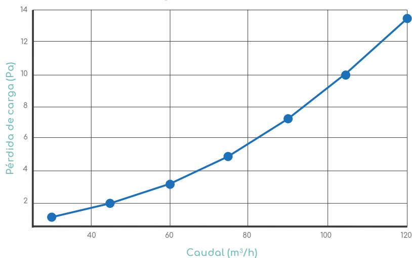
Pérdida de carga vs Caudal de salida 3 x Ø 75
